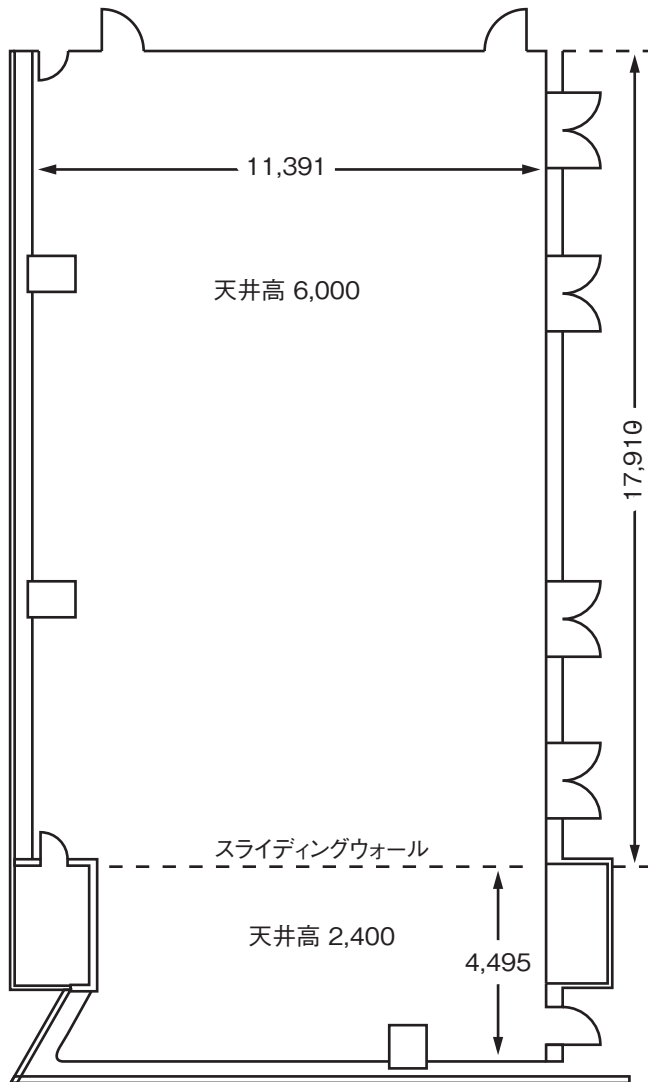
平面図
